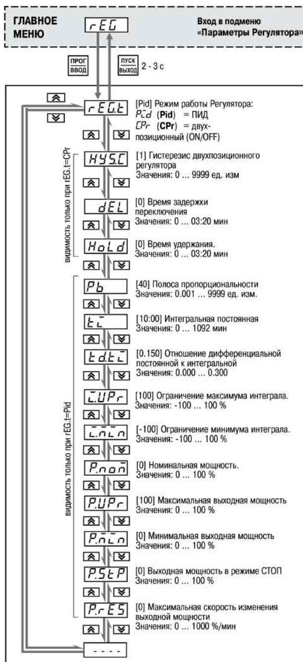
Рисунок 8.3 – Параметры регулятора
